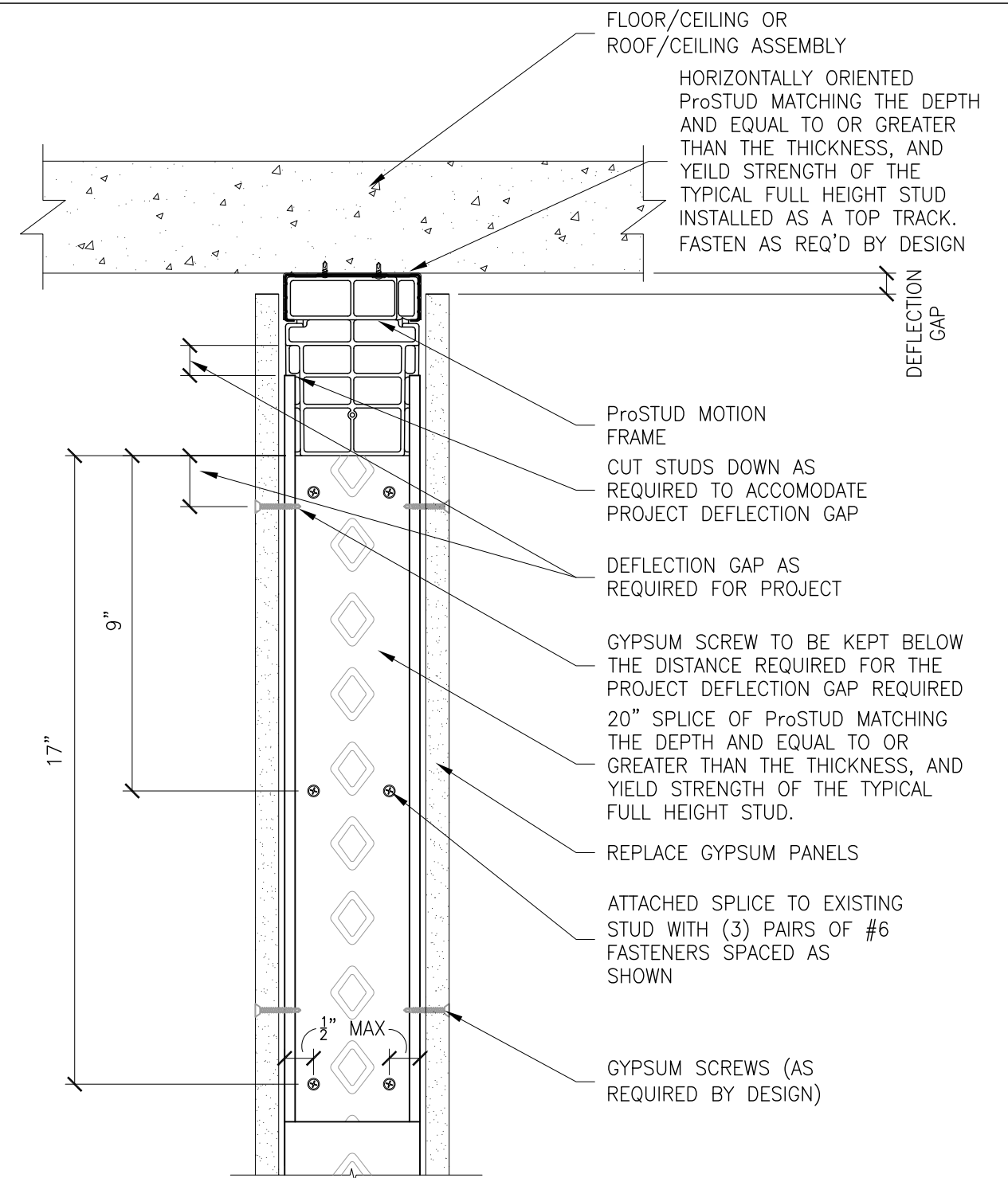
SECTION A-A
