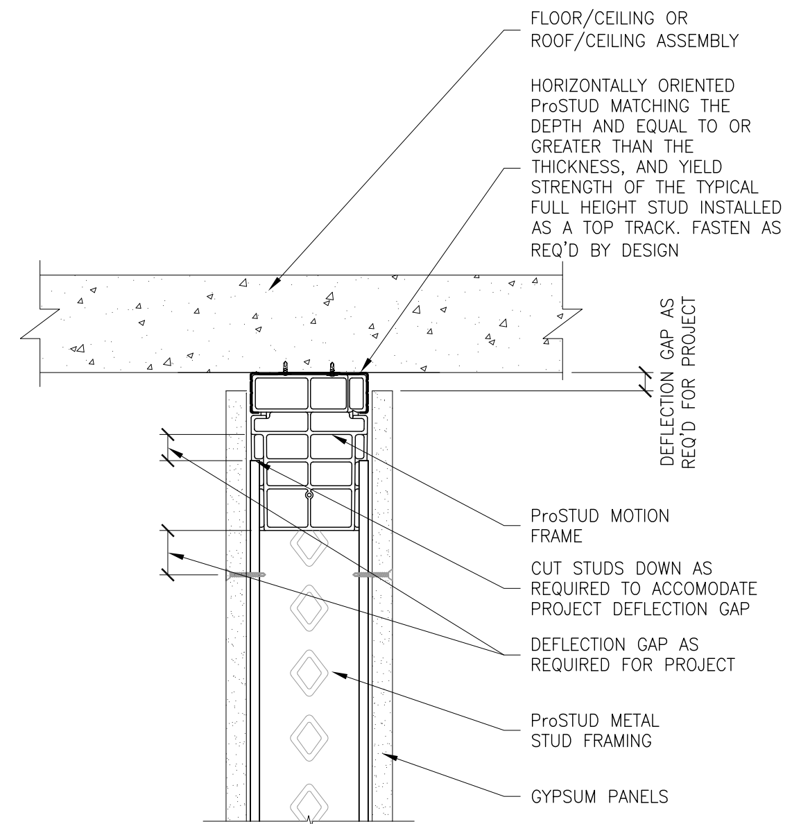
SECTION A-A
